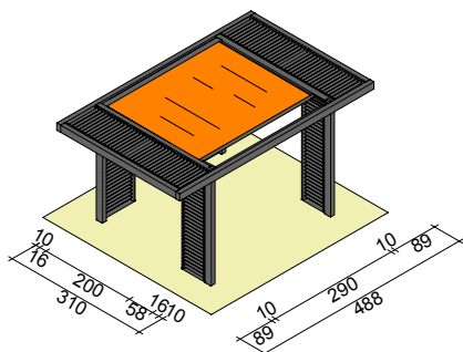
Pergola indipendente Kronos
