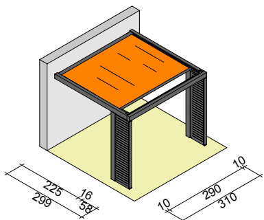
Pergola addossata Kronos
