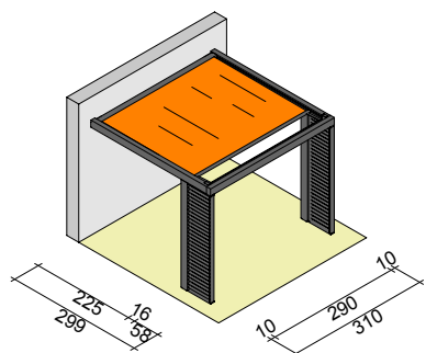
Pergola addossata Kronos
